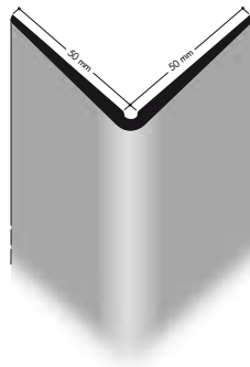
Profilo parabordi e paraspigoli nora ® K 9022
